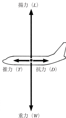
◀ 図1-5 水平定常飛行中の力のつり合い
